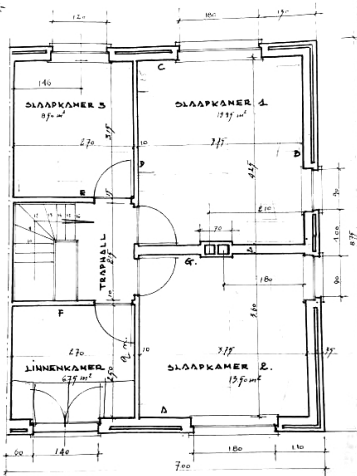
— PLAN VERDIEPING —
