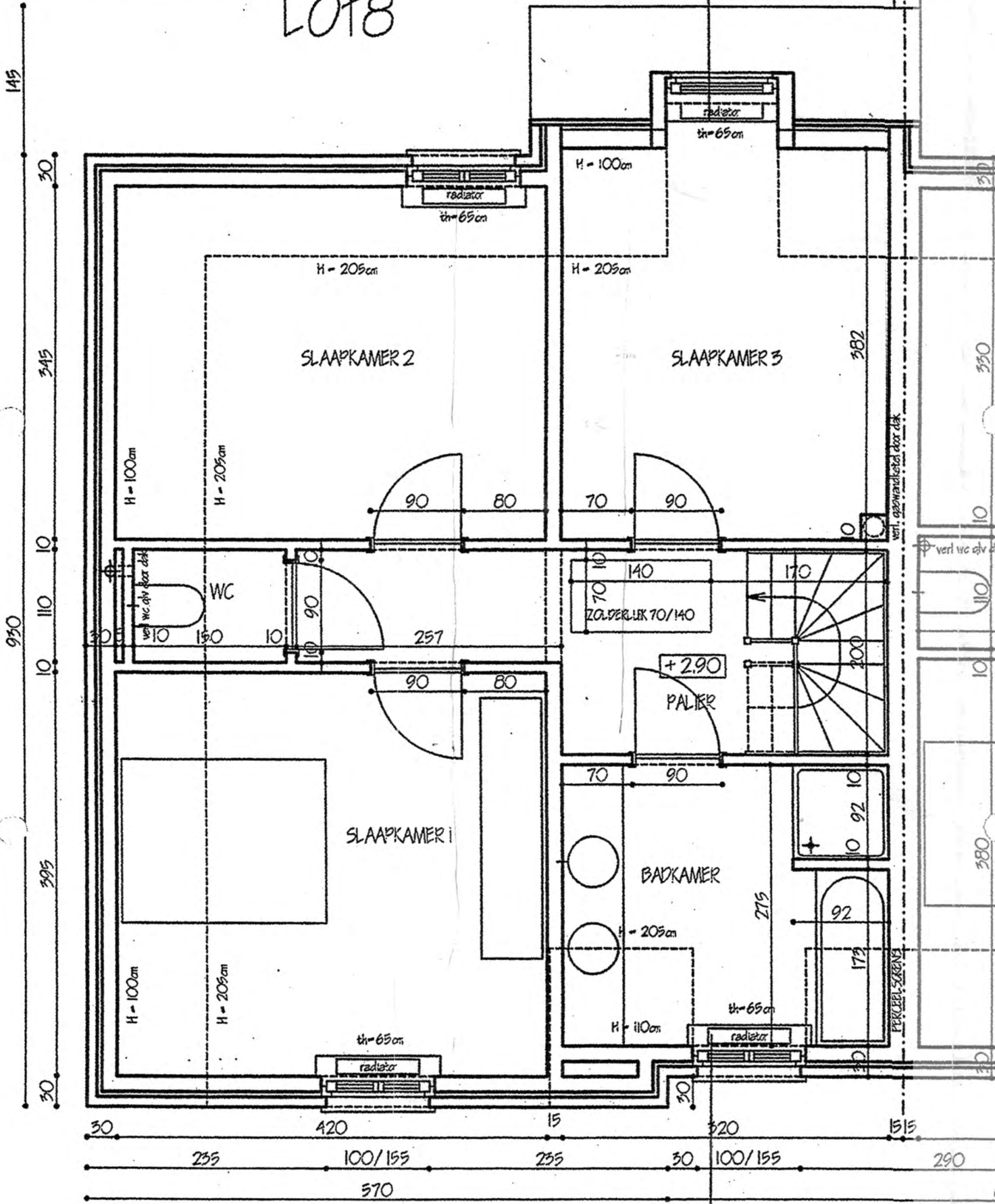
VERDIEPINGSPLAN
